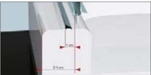
Installazione e ingombro del frangiflutto.
